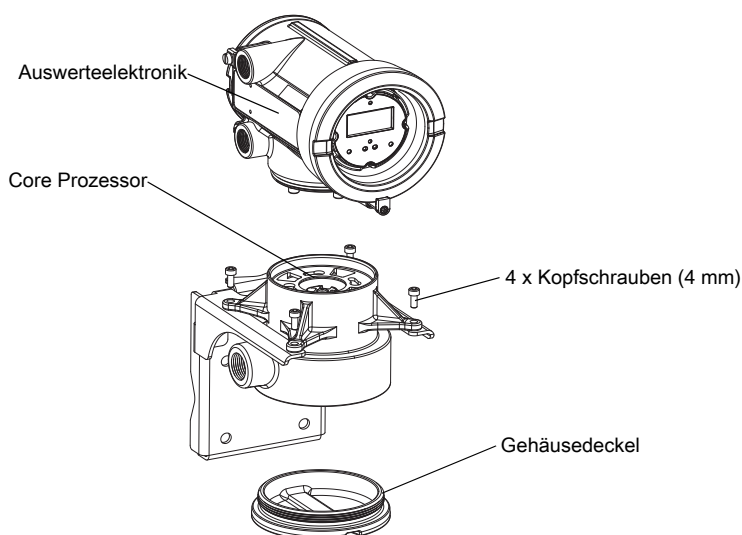
Abbildung 10-2: 9-adrige Installationskomponenten
