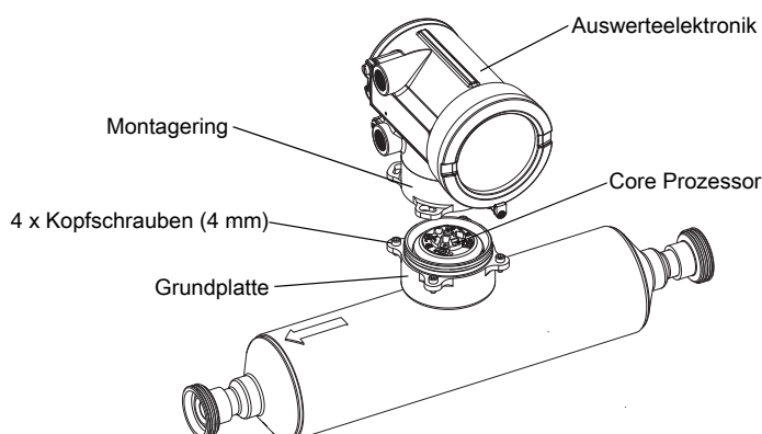
Abbildung 10-3: Komponenten der integrierten Installation
