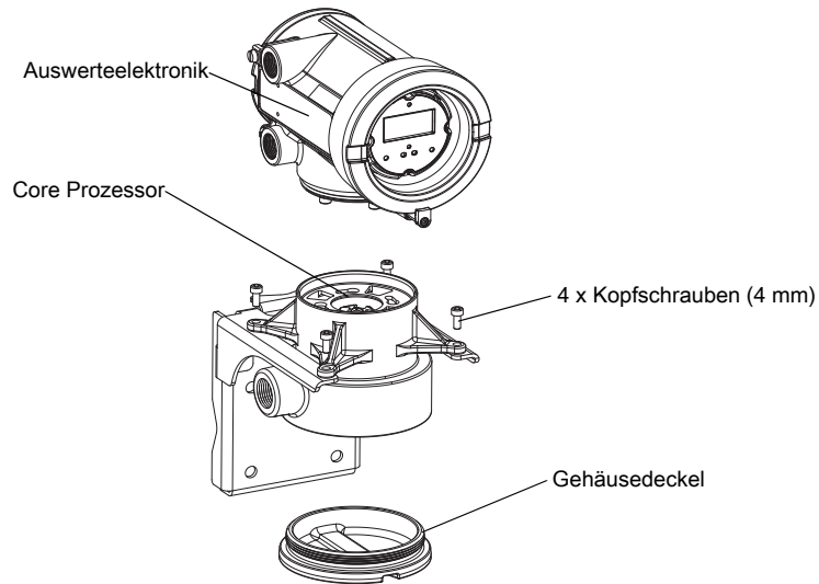
Abbildung 10-4: 9-adrige Installationskomponenten
