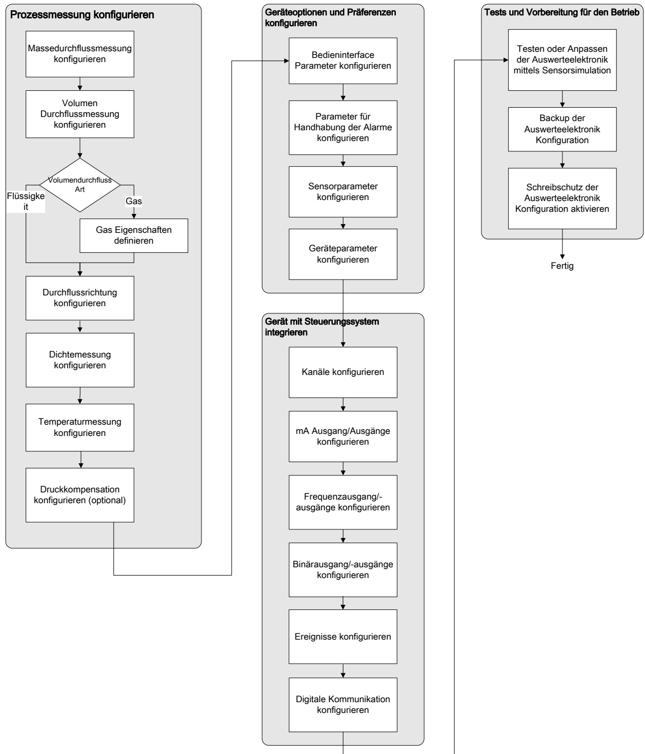
Abbildung 3-1: Ablaufdiagramm - Konfiguration
